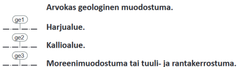
Kuva 7: Arvokkaan geologisen muodostuman kaavamerkintä Pirkanmaan maakuntakaava 2040:ssä.
